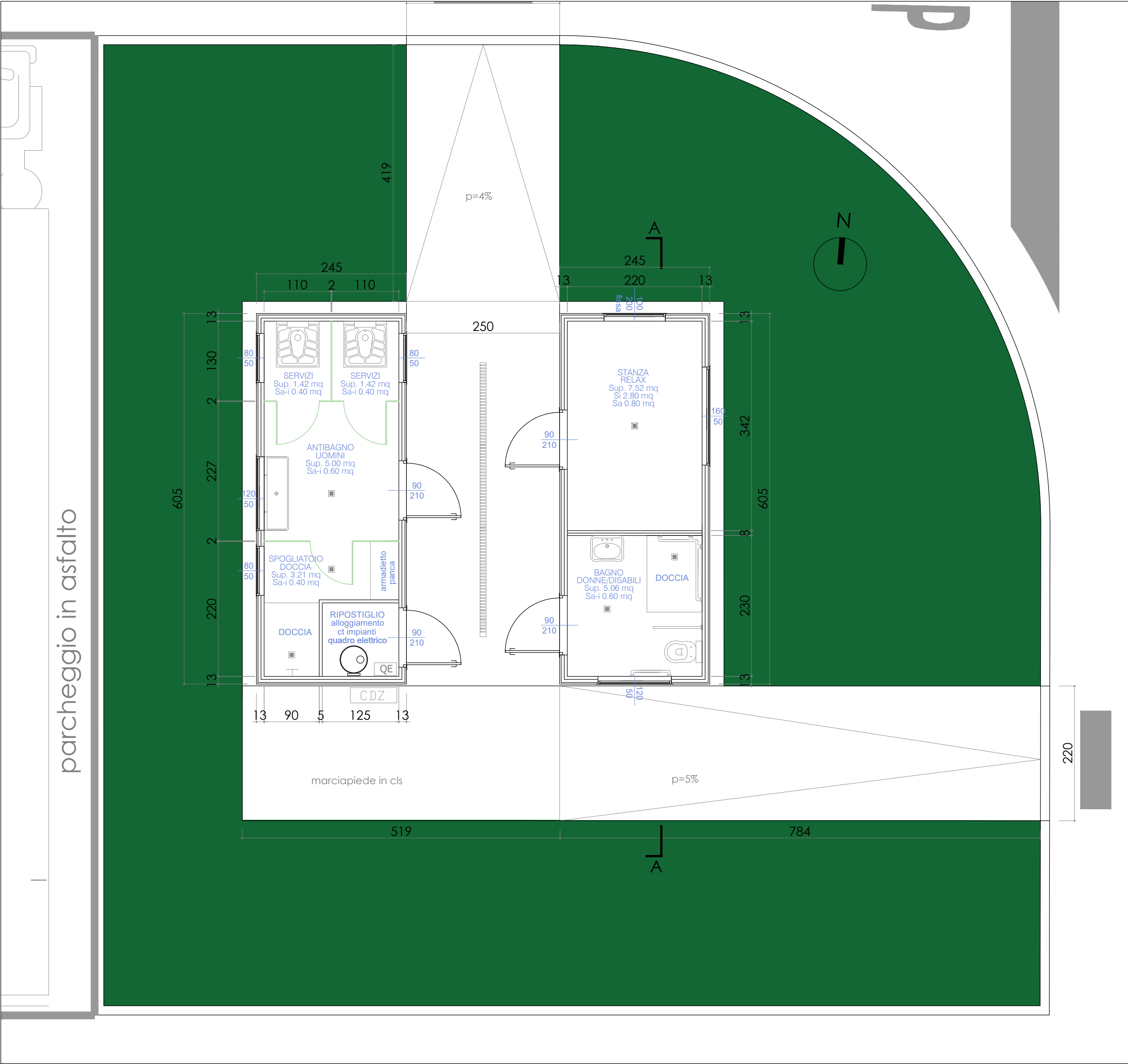
pianta scala 1:50
