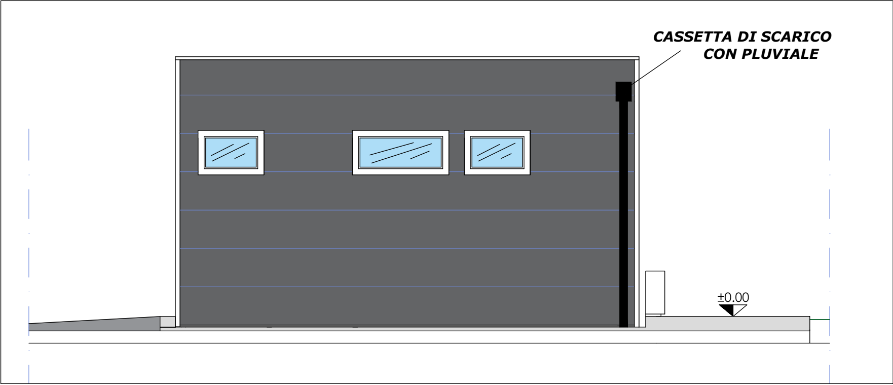
prospetto ovest scala 1:50
